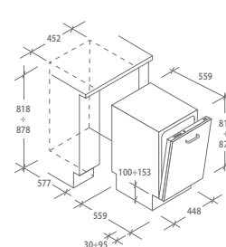
ESQUEMA (mm)
