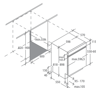
ESQUEMA (mm)
